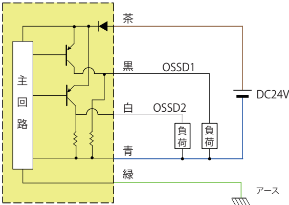
PNP出力回路
