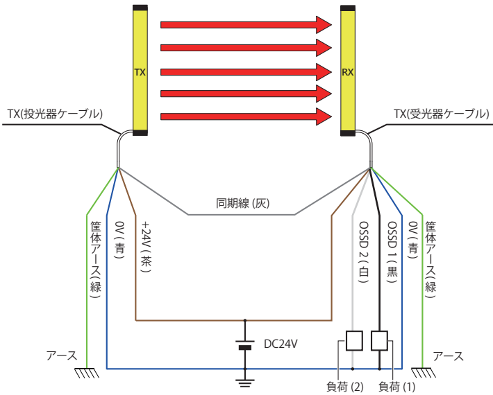
PNP出力回路
