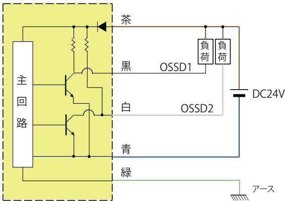
NPN出力回路
