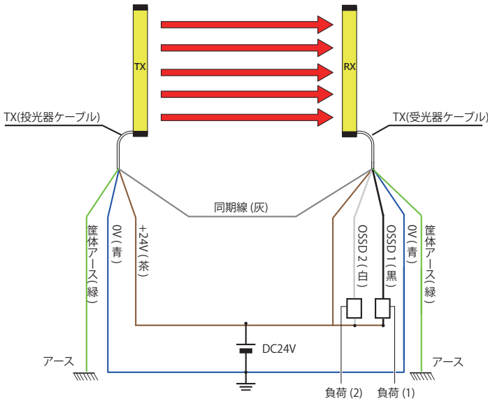
NPN出力回路
